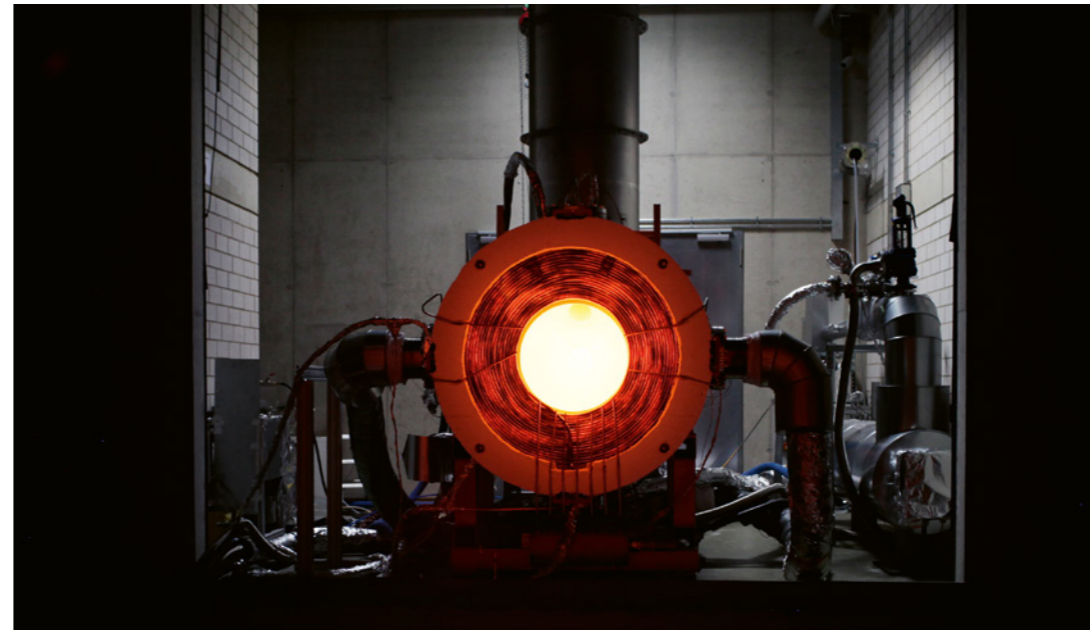
Test der 200-kW-Pilotanlage unter künstlicher Sonne am DLR Synlight in Jülich
